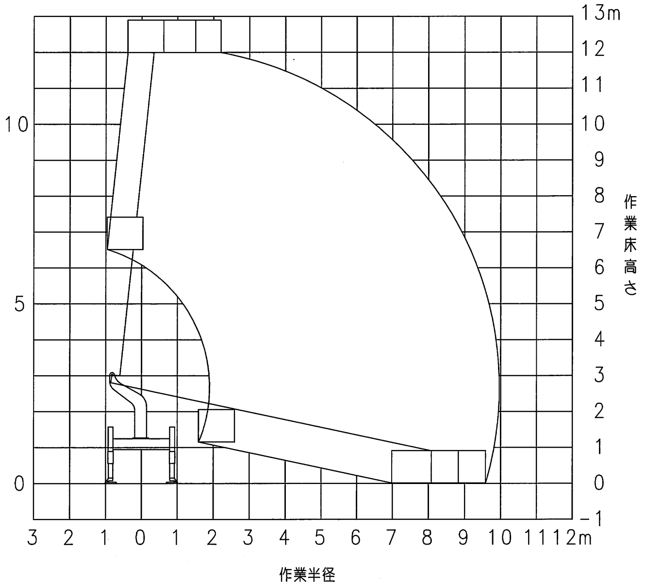
図1 作業範囲図
