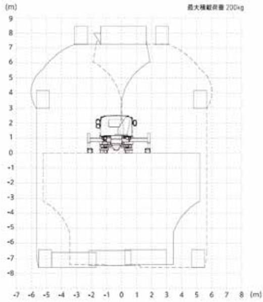
アウトリガー張出幅 最大 (左側 1.81~1.84 右側 2.14~2.17) ※車体中心から
