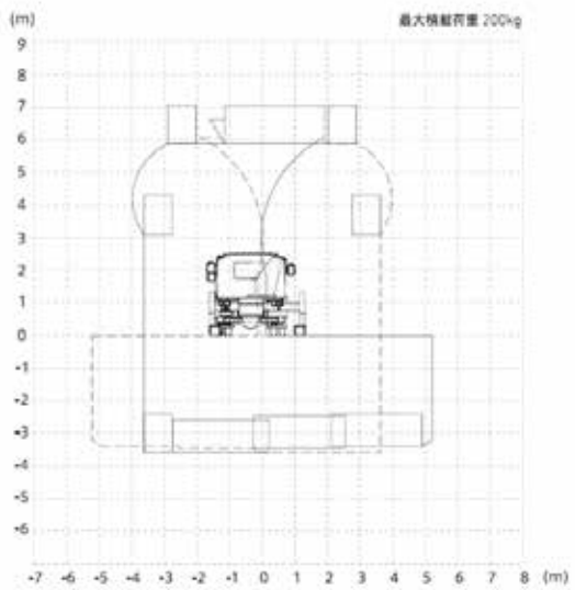
アウトリガー張出幅 最小 (左側 1.15~1.38 右側 1.56~1.77) (左側のみ作業可能) ※車体中心から
