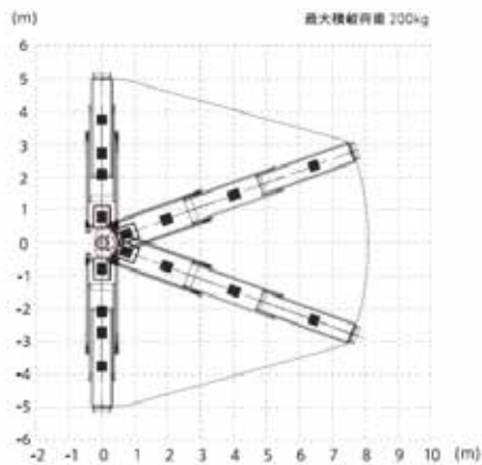
アウトリガー張出幅 格納 (左側 1.01~1.15 右側 1.01~1.56) プラットフォーム作業範囲図 ※車体中心から
