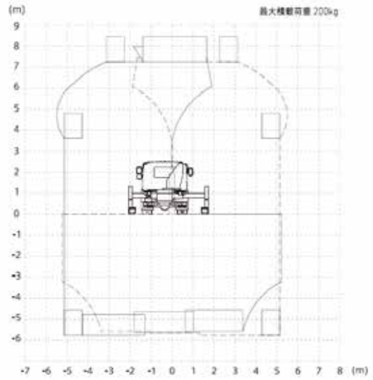
アウトリガー張出幅 中間2 (左側 1.61~1.61 右側 1.97~2.14) ※車体中心から
