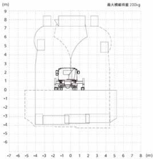
アウトリガー張出幅 中間1 (左側 1.38~1.61 右側 1.77~1.97) ※車体中心から
